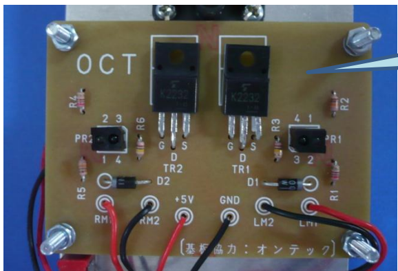
半田付け部分以外は レジストがあるので 半田付け失敗の心配 なし
